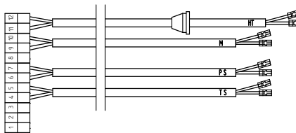
Кабель X5 (комплект) - 3414358 (solo turbo)
