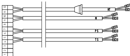
Кабель X5 (комплект) - 3414358 / СТ
