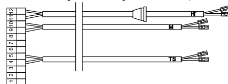
Кабель X5 (комплект) - 3414358 / СТ
