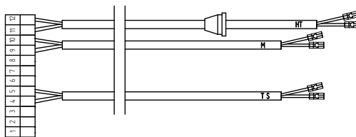
Кабель X5 (комплект) - 3414358 (solo turbo)
