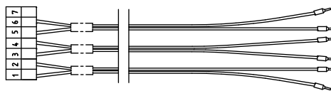
14. Кабель X3 (комплект) - 3414348
