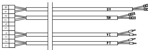
16. Кабель X6 (комплект) - 3414350 (комби турбо)
