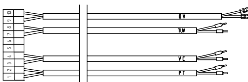
Кабель X6 (комплект) - 3414357 / СТ, СК
