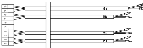
Кабель X6 (комплект) - 3414357 (solo turbo)
